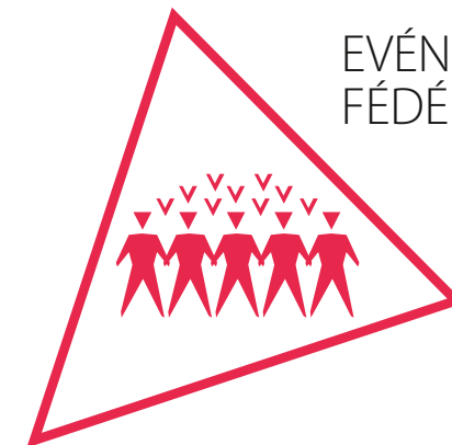
ECOSYSTÈME DYNAMIQUE
